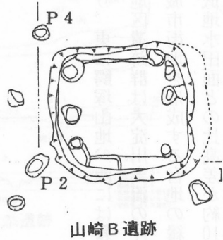
第2図 各遺跡の竪穴建物跡（鹿児島県）
