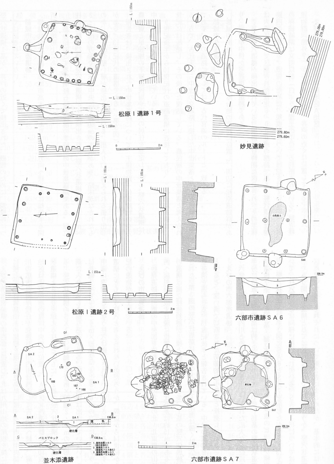
第3図 各遺跡の竪穴建物跡 (宮崎県)
