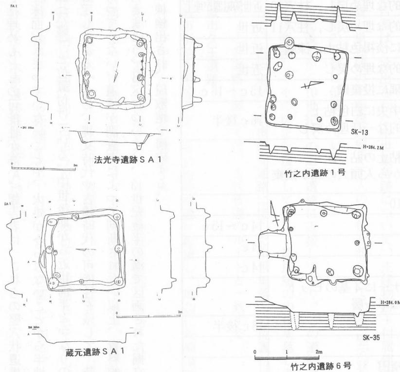
第4図 各遺跡の竪穴建物跡（宮崎県）
