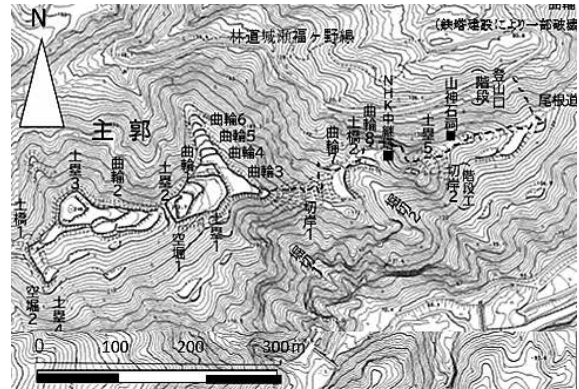
図2 狩集陣跡実測平面図
