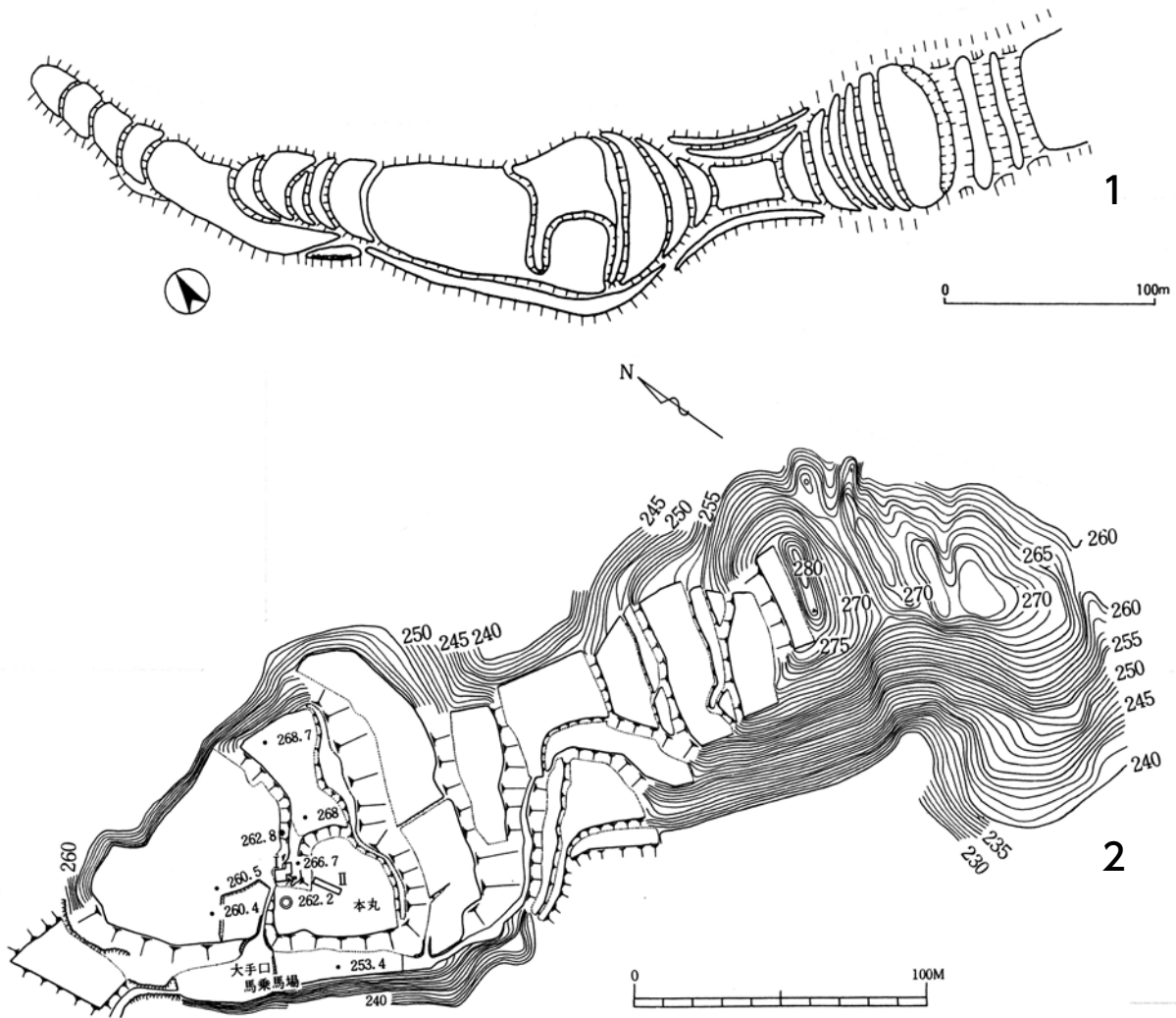
第2図 廻城跡縄張り図・測量図
